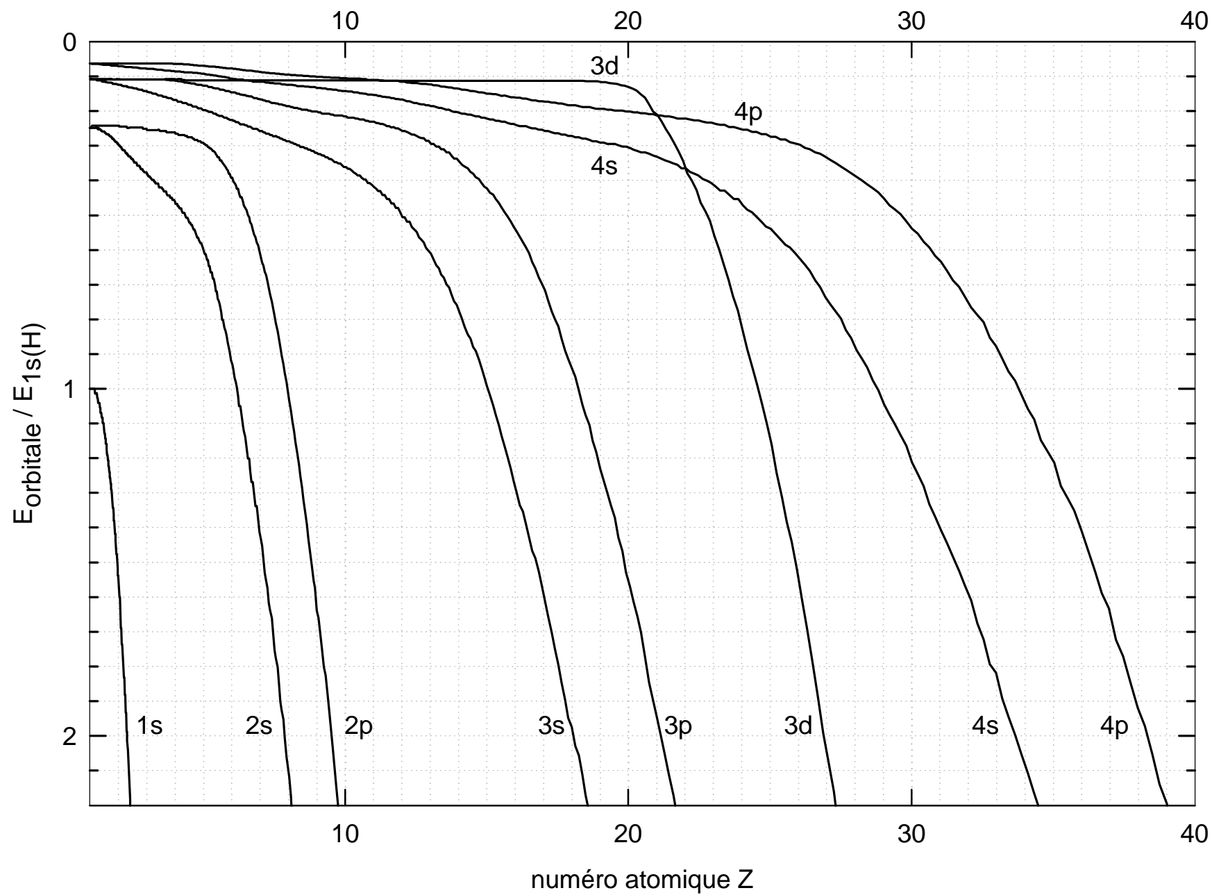
Énergie des orbitales dans les atomes polyélectroniques neutres en fonction de la charge du noyau ( E_{1s(H)} = -13.59\text{eV} )
